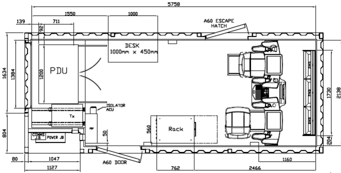
ROV Control Van
